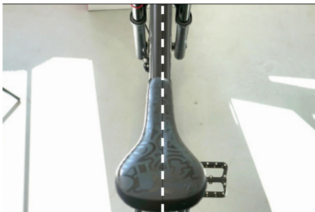
Afbeelding 45: Zadel in rijrichting uitlijnen
